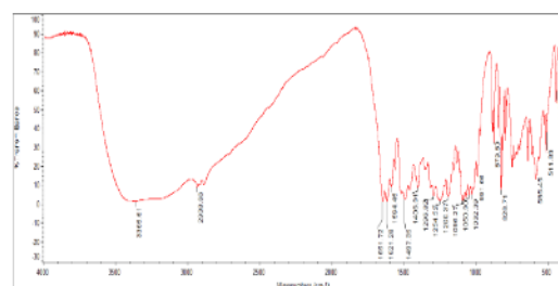
Fig. 3. IR Spectrum of Mangiferin
